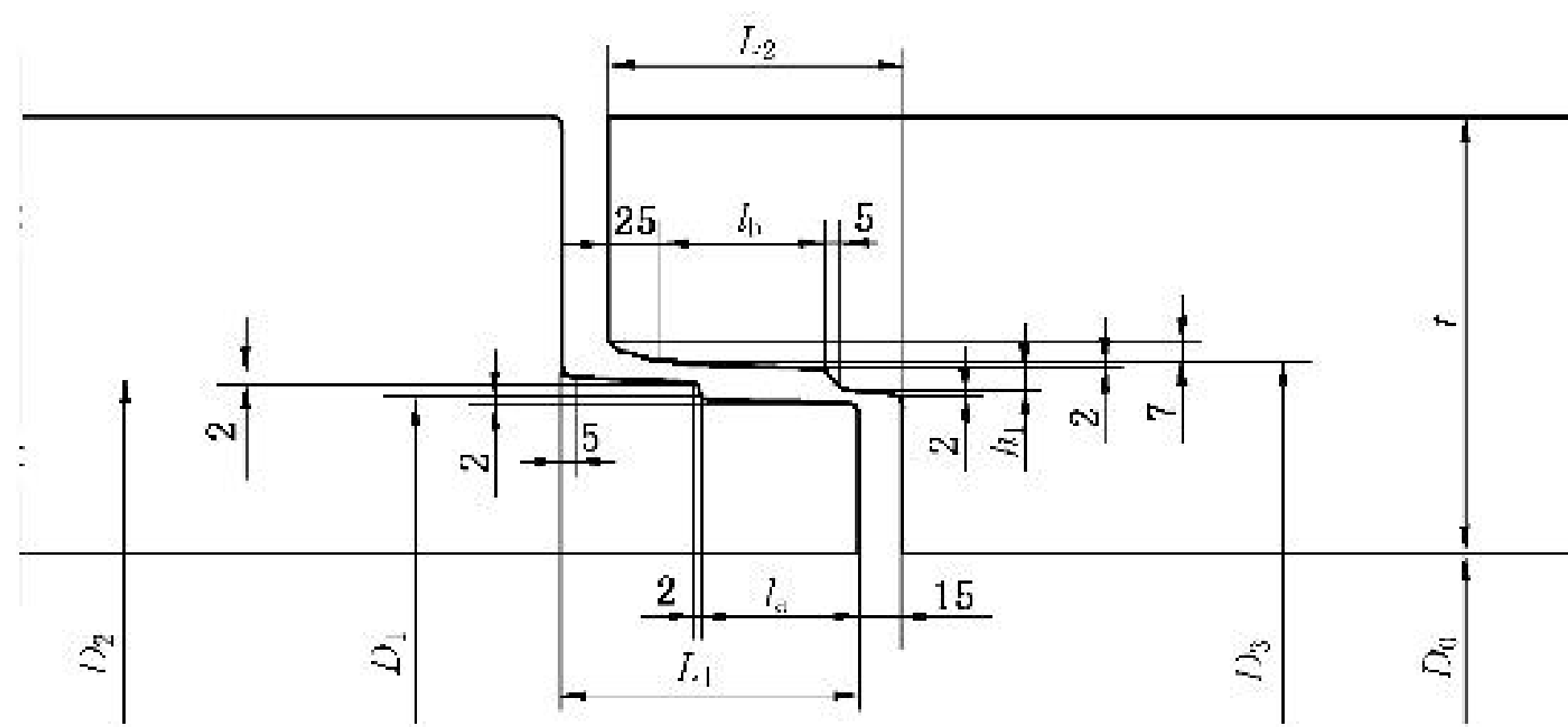
a) \phi 1\ 350\sim\phi 4\ 000 柔性接口 A 型企口管接口
