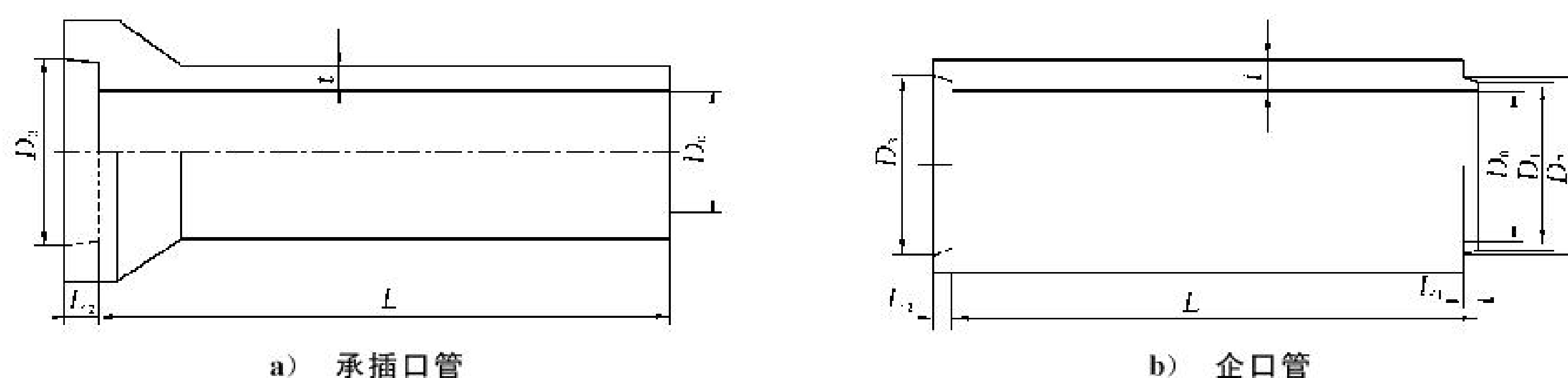
图 1 柔性接口管外形示意图（续）
