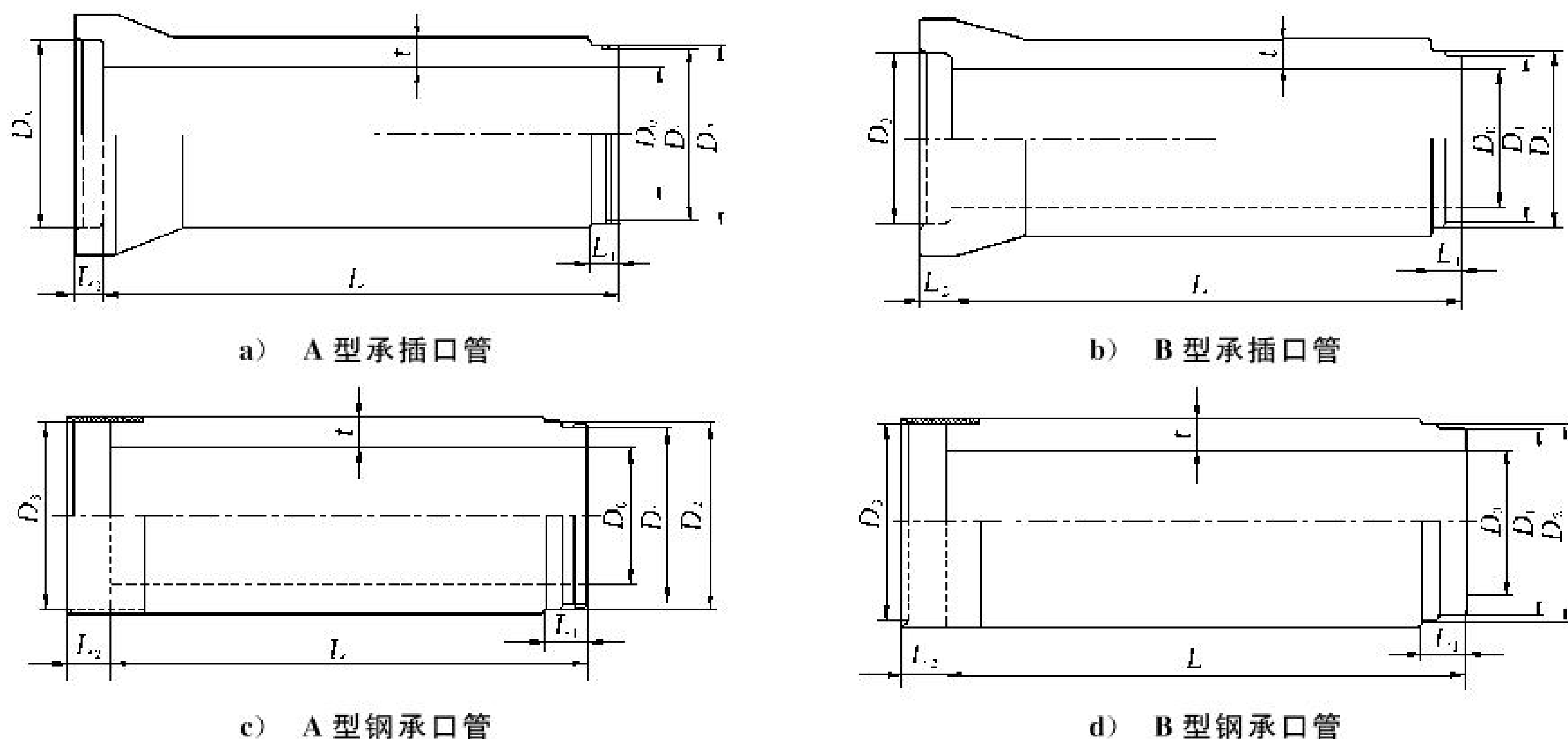
图 1 柔性接口管外形示意图
