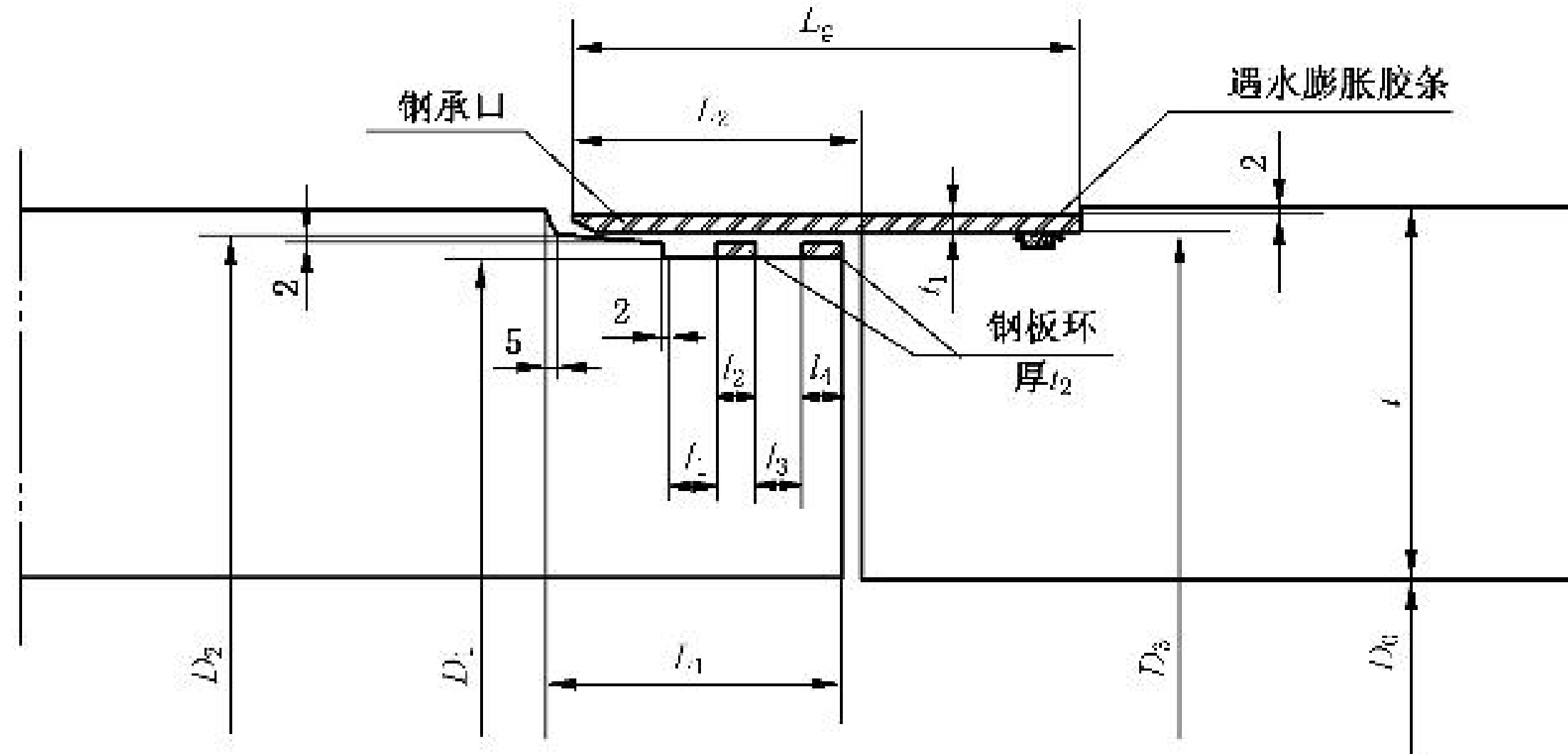
图 A.7 \phi 800 \sim \phi 4\,000 柔性接口 D 型钢承口管接口
